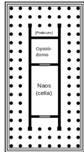
DÍPTERO
